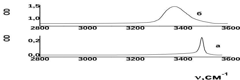
Расми 2 . Спектрҳои инфрасурхи таҷрибавии мономери имидазол (а) ва Н-комплексҳои он бо атсетонитрил (б) дар ҳудуди лапишҳои валентии N–H.
