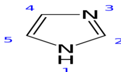
Расми 1. Сохтори молекулаи имидазол.
