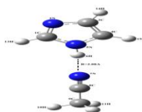
Расми 4. Сохтори бавуҷудии алоқаҳои гидрогени байнимолекулии имидазол бо ацетонитрил.
