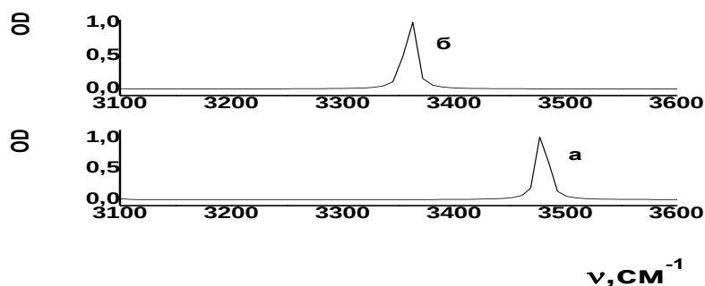
Расми 3. Спектрҳои инфрасурхи назариявии мономери имидазол (а) ва Н-комплексҳои он бо атсетонитрил (б) дар ҳудуди лапишҳои валентии N–H
