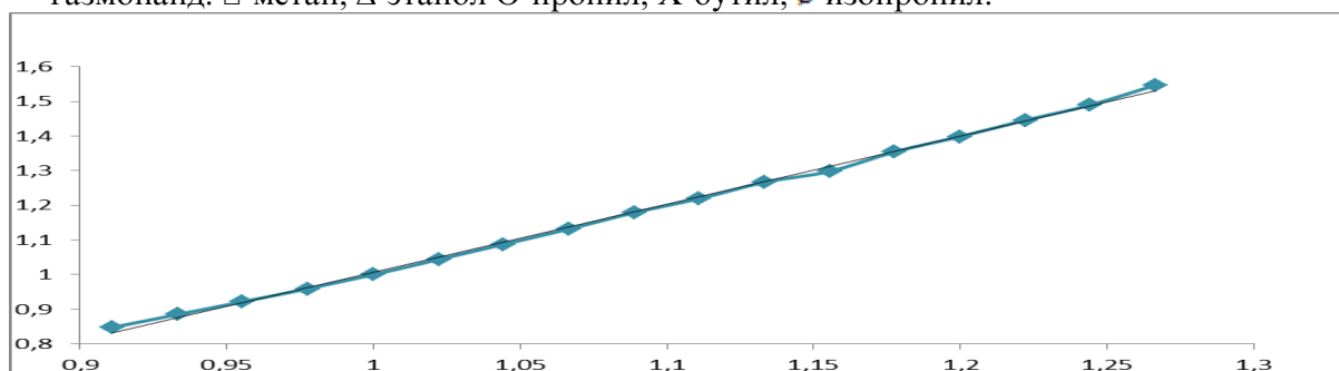
Расми 2. Гармигузаронии спирти метил вобаста ба ҳарорат T, K.
