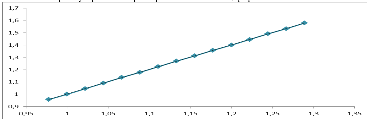
Расми 5. Гармигузаронии спирти дибутил вобаста ба ҳарорат.
