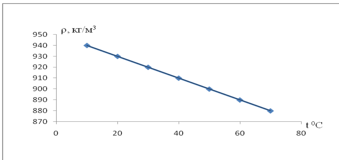
Расми 1: Вобастагии зичии рағани зағир аз ҳарорат
