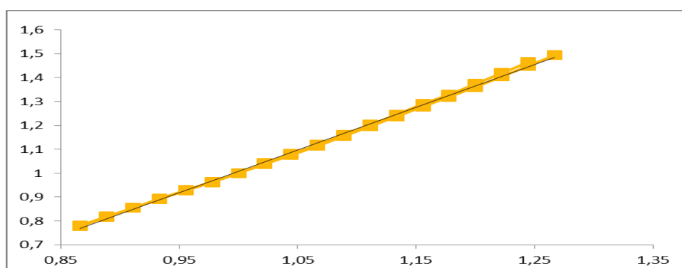
Расми 1. Вобастагии \lambda/\lambda_1 аз ҳарорати овардашуда T/T_1 барои спиртҳои газмонанд: □-метан; Δ-этанол О-пропил; X-бутил; ○-изопропил.
