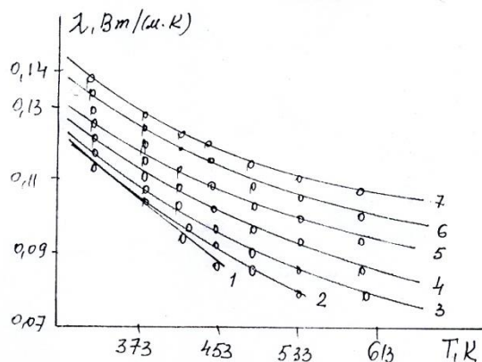
Расми 3. Изобараҳои коэффисенти гармигузаронии Н-гексан: 1-0,098; 2- 4,9; 3- 9,8; 4 – 19,6; 5 – 29,4; 6 – 39, 7 – 49,0 МПа. Расми 4. Изобараҳои коэффисенти гармигузаронии Н-гексан-1: 1-0,098; 2- 4,9; 3- 9,8; 4 – 19,6; 5 – 29,4; 6 – 39,2; 7 – 49,0 МПа
