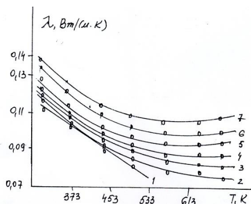
Расми 3. Изобараҳои коэффисенти гармигузаронии Н-гексан: 1-0,098; 2- 4,9; 3- 9,8; 4 – 19,6; 5 – 29,4; 6 – 39, 7 – 49,0 МПа. Расми 4. Изобараҳои коэффисенти гармигузаронии Н-гексан-1: 1-0,098; 2- 4,9; 3- 9,8; 4 – 19,6; 5 – 29,4; 6 – 39,2; 7 – 49,0 МПа
