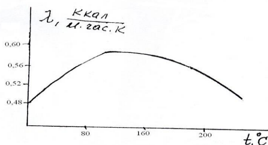
Расми 1. Вобастагии гармогузаронии об аз ҳарорат
