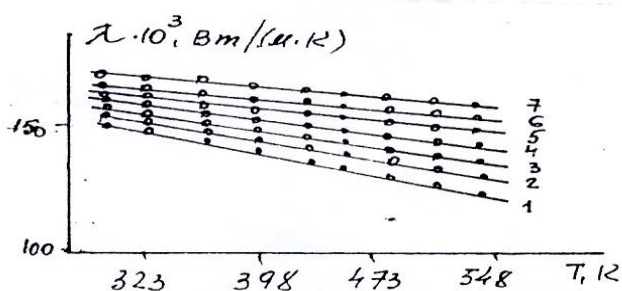
Расми 2. Гармигузаронии дипропилфталати моеъ вобаста аз ҳарорат ва фишор ( 10^5 \text{ Па} ): 1-0,98; 2-4,9; 3-9,8; 4-19,6; 5-29,4; 6-39,3; 7-49,0.
