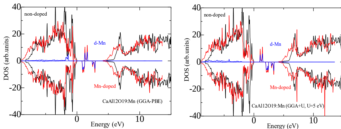
Рис. 1. Плотность электронных состояний \text{CaAl}_{12}\text{O}_{19}:\text{Mn}^{4+} по GGA и GGA+U ( U=5\text{ эВ} ) расчетам.
